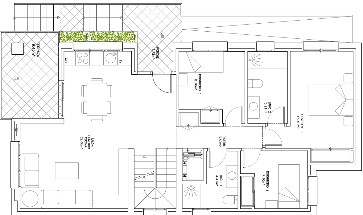
PLANTA BAJA
