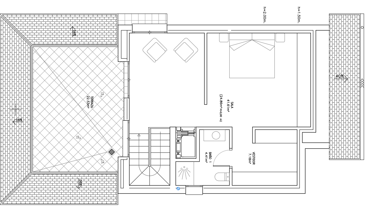
PLANTA ALTA
